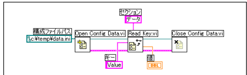
図 13-6 .ini ファイルからのデータの読み取り
