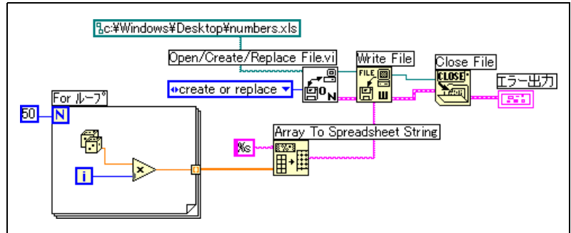
図 13-2 低レベル VI によるスプレッドシートへの書き込み
