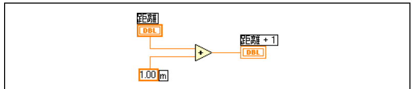
図 5-7 単位を持つ増分関数の作成
