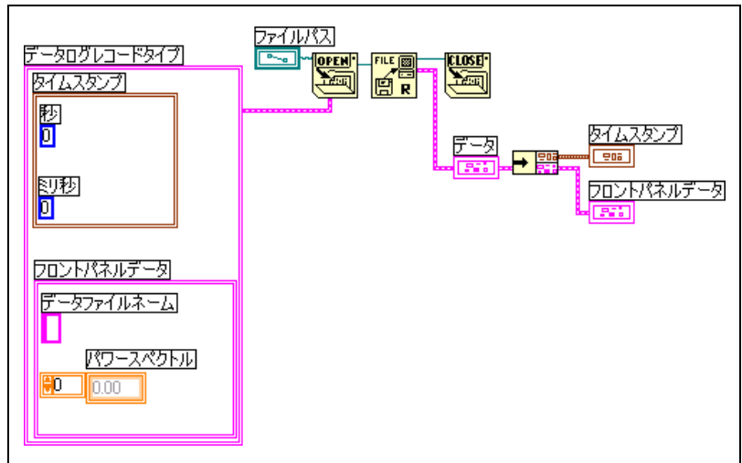
図 13-10 File Open 関数を使用した記録済みデータの取り出し
