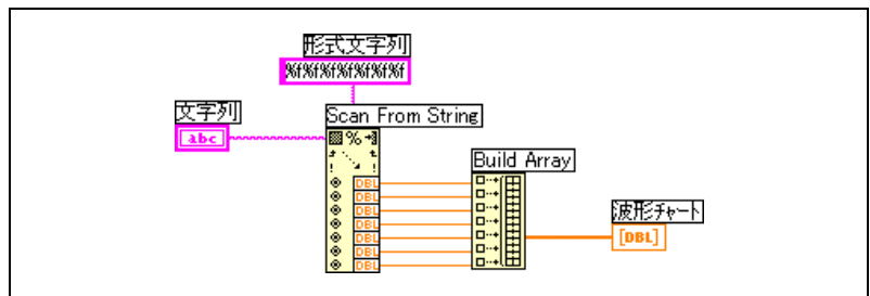
図 9-2 文字列を数値に変換する
