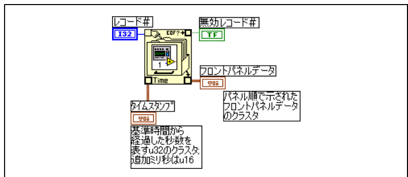
図 13-8 記録済みデータの取り出し
