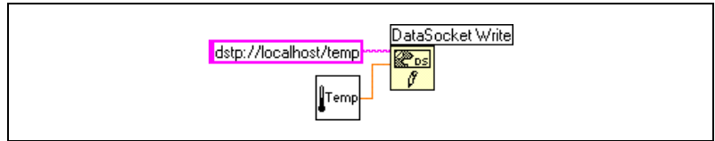
図 17-1 DataSocket Write を使用してデータをパブリッシュする
