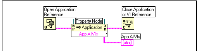
図 16-1 ローカルコンピュータ上のメモリ内の VI をすべて表示する
