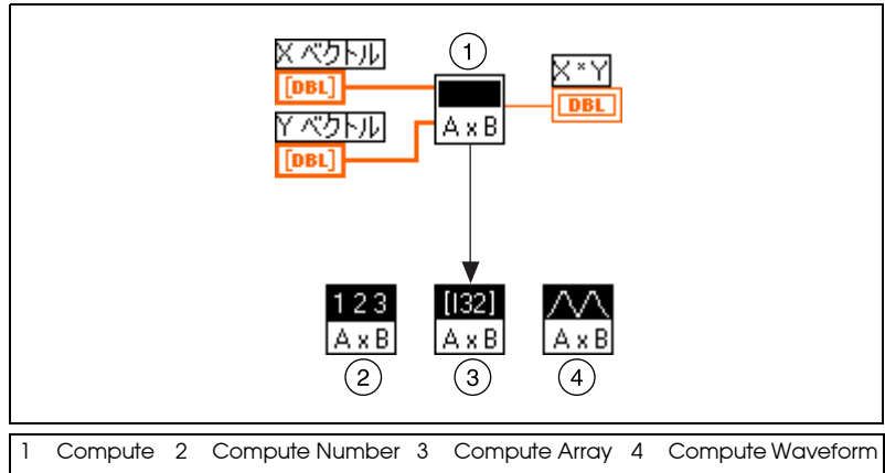
図 5-3 サブ VI を呼び出す多形性 VI
