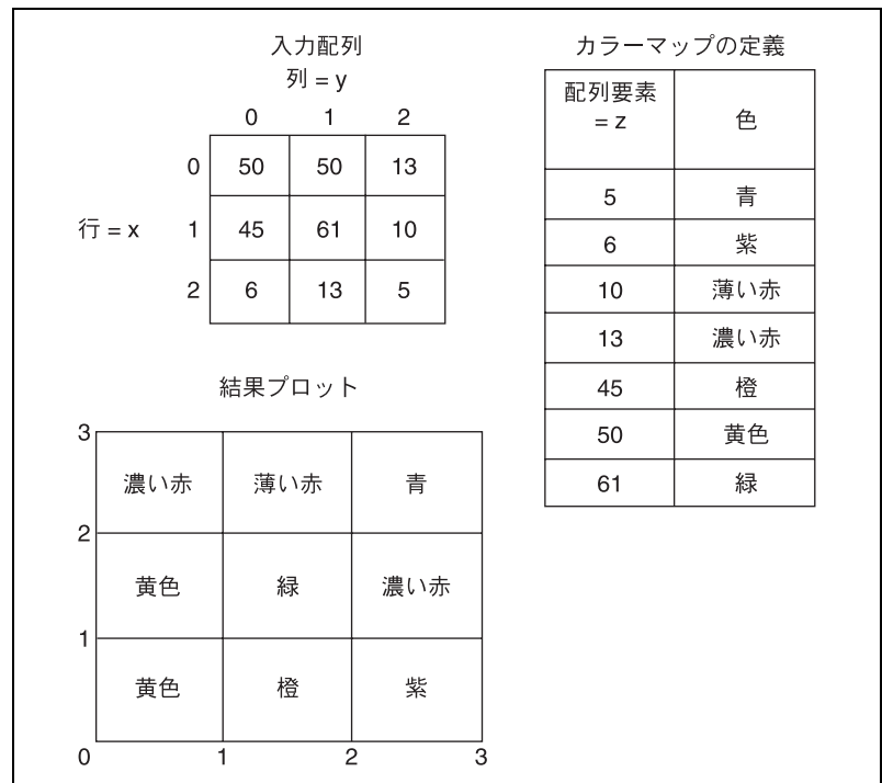
図 11-5 強度チャートのカラーマップ
