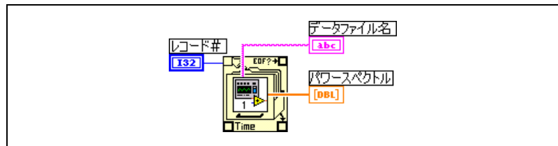
図 13-9 サブ VI の端子を経由した記録済みデータの取り出し
