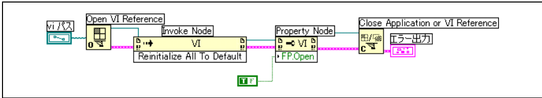
図 16-3 VI クラスのプロパティとインボークノードを使用する
