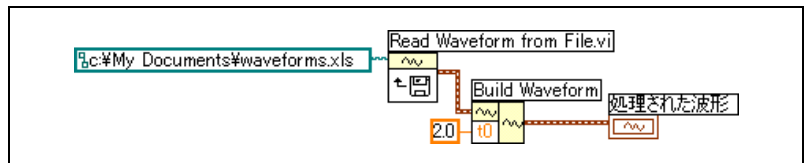
図 13-4 ファイルからの波形の読み取り
