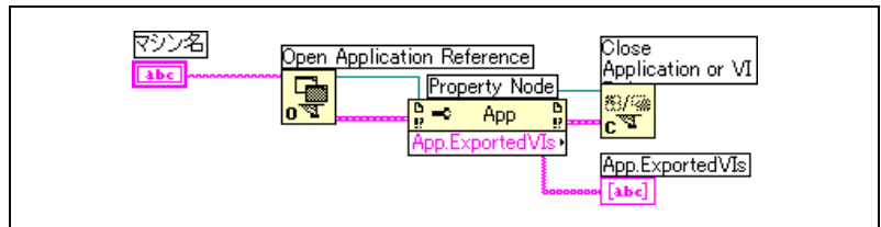
図 16-2 リモートコンピュータ上のメモリ内の VI をすべて表示する
