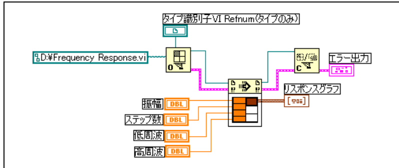
図 16-5 Call By Reference Node を使用する
