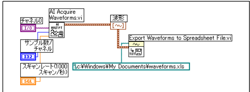
図 13-3 スプレッドシートファイルへの複数の波形の書き込み
