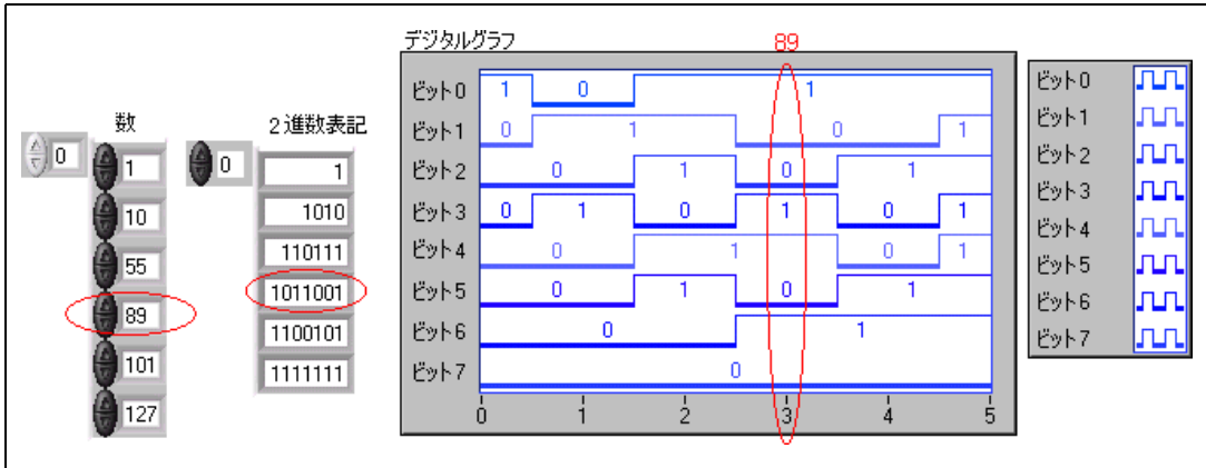
図 11-6 デジタル形式での整数のグラフ化
