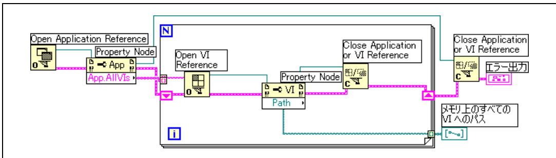
図 16-4 アプリケーションおよび VI クラスのプロパティとメソッドを使用する
