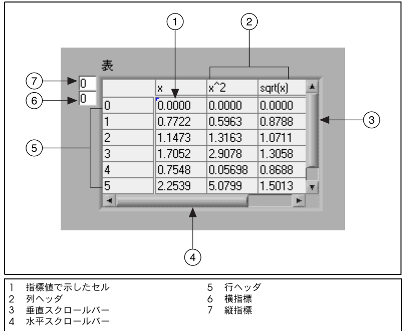
図 9-1 表の構成要素
