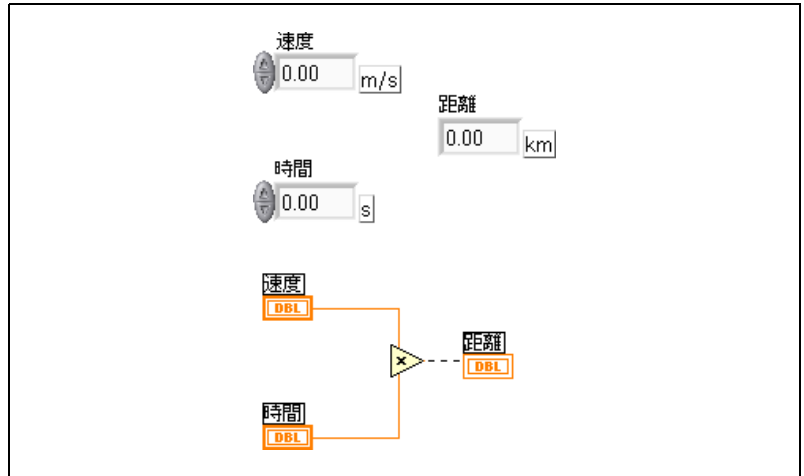
図 5-6 単位に互換性がないオブジェクトの配線により壊れたワイヤ
