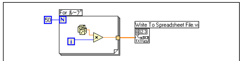
図 13-1 高レベル VI によるスプレッドシートへの書き込み
