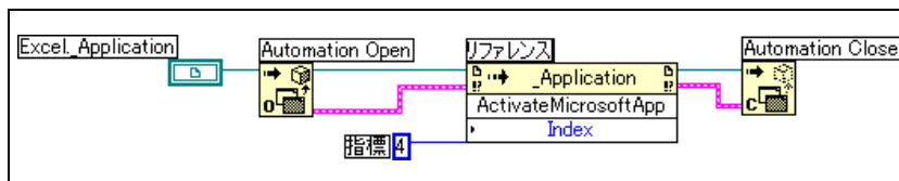
図 18-2 数値定数でデータ値を設定する
