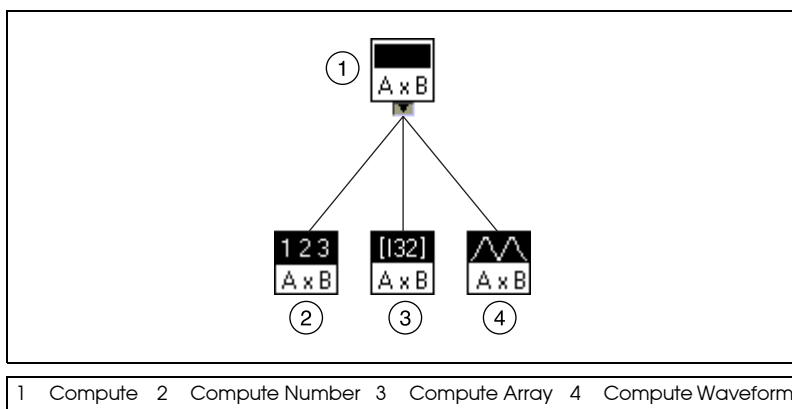
図 5-2 多形性 VI の例
