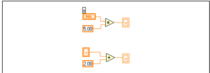
図 10-1 競合状態
