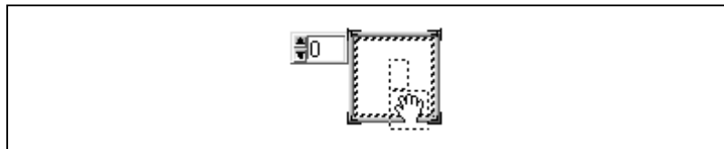
図 9-7 配列シェル
