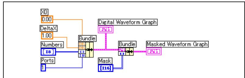
図 D-1 デジタルデータをマスクする
